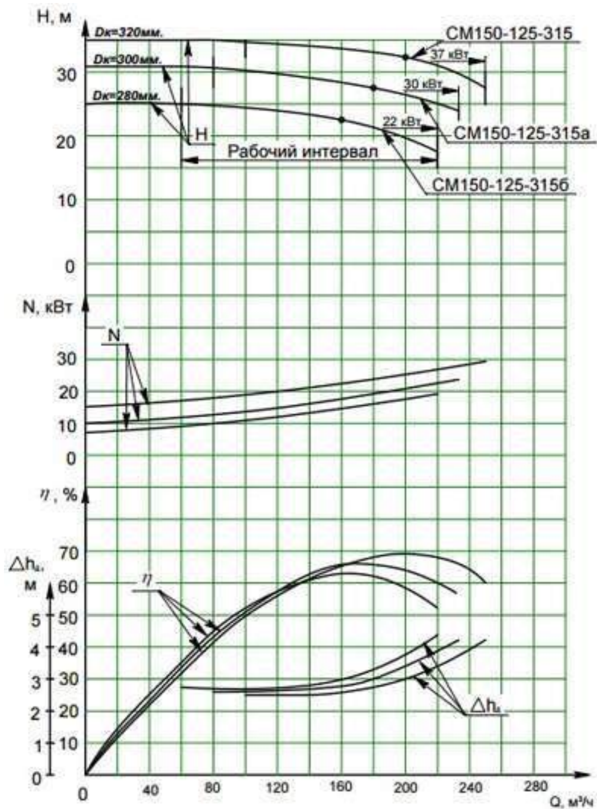
Рисунок 3.3.4.1 - Гидравлические характеристики насосов CM 150-125-315/4
