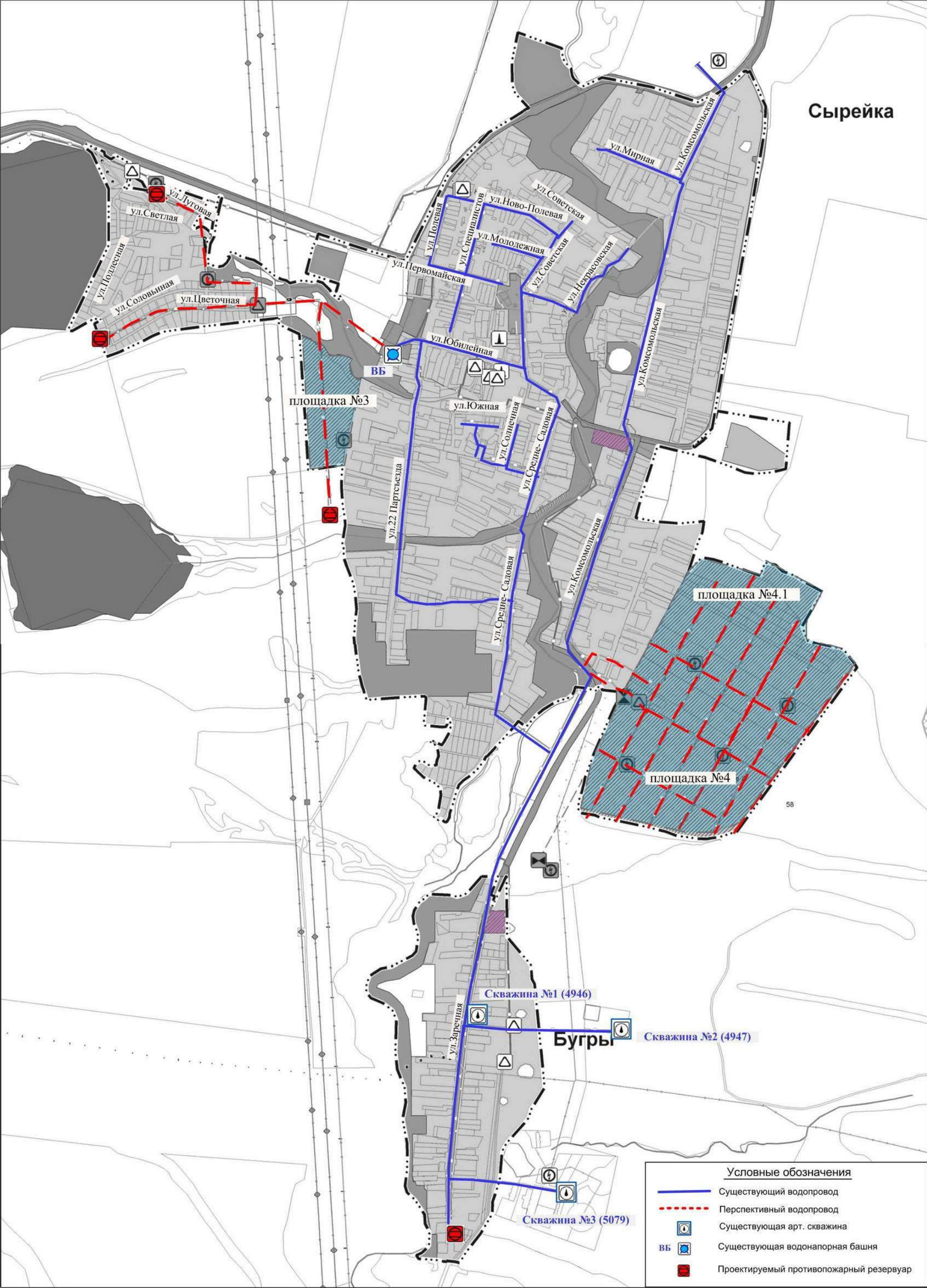
Рисунок 2.4.9.2 - План развития централизованных систем водоснабжения с. Сырейка, п. Бугры
