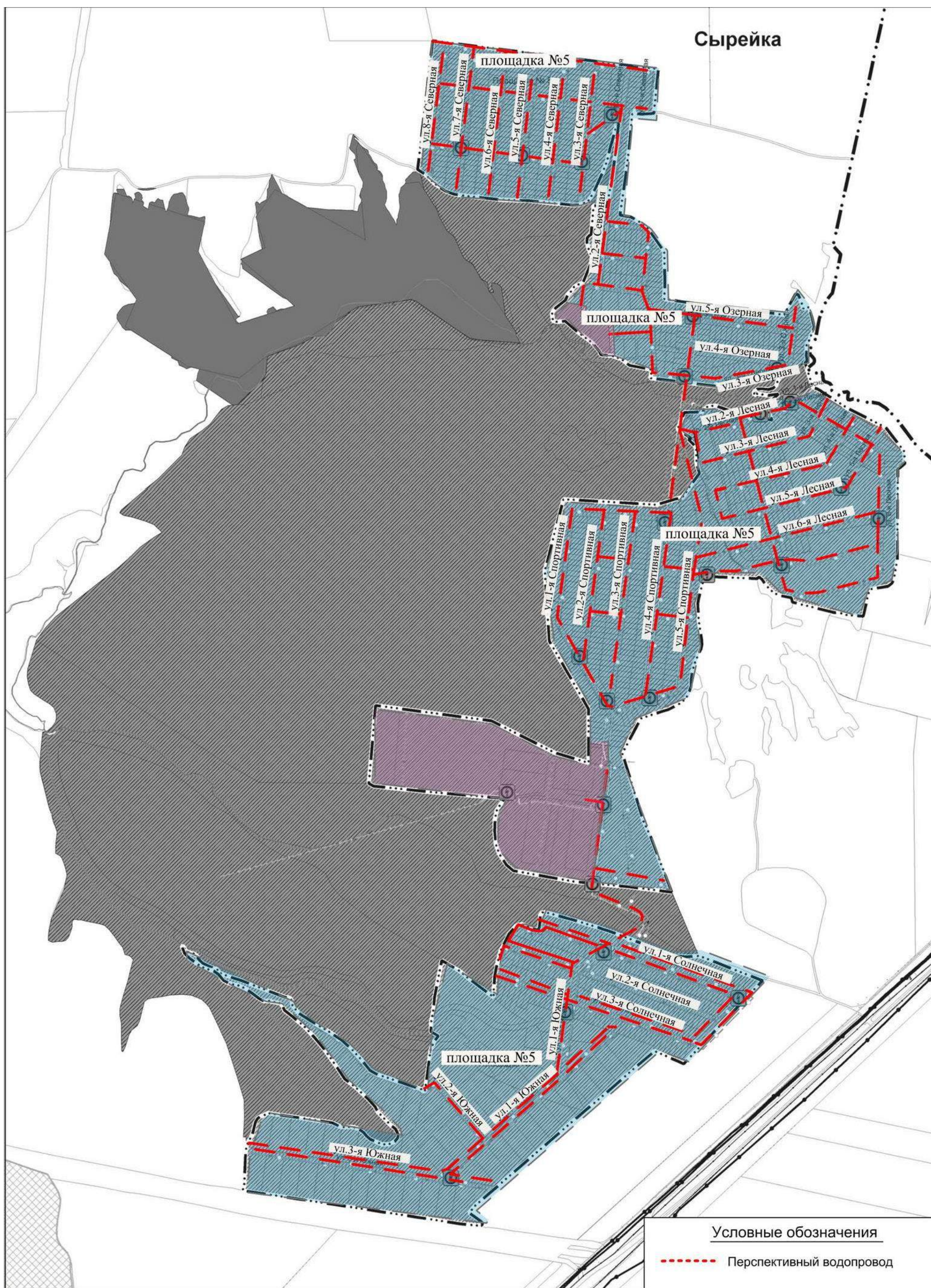
Рисунок 2.4.9.3 - План развития централизованных систем водоснабжения на площадке №5 с. Сырейка
