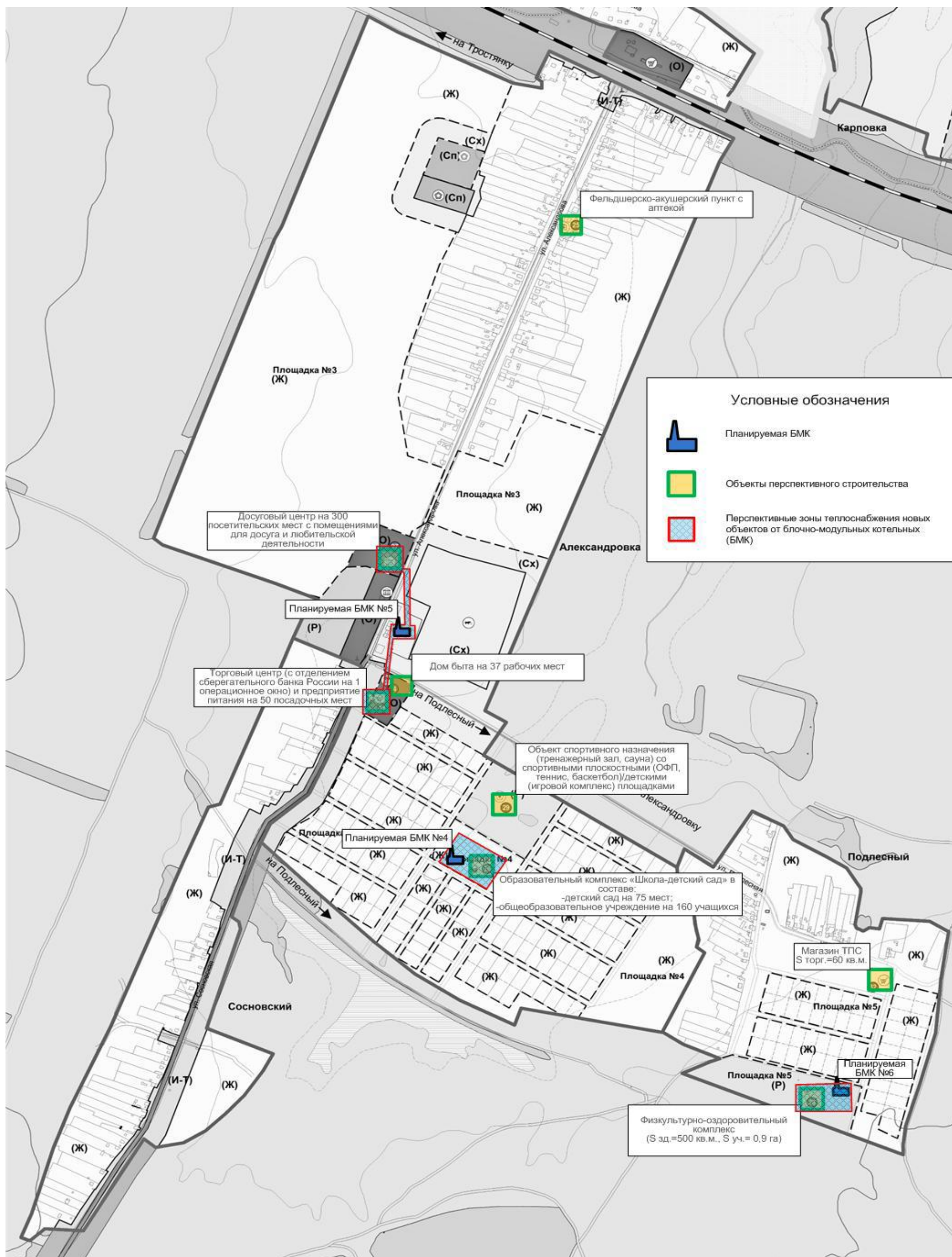
Рис. № 13 – Перспективные зоны теплоснабжения планируемых блочно-модульных источников тепловой энергии, планируемых к размещению на территории села Александровка и поселка Подлесный
